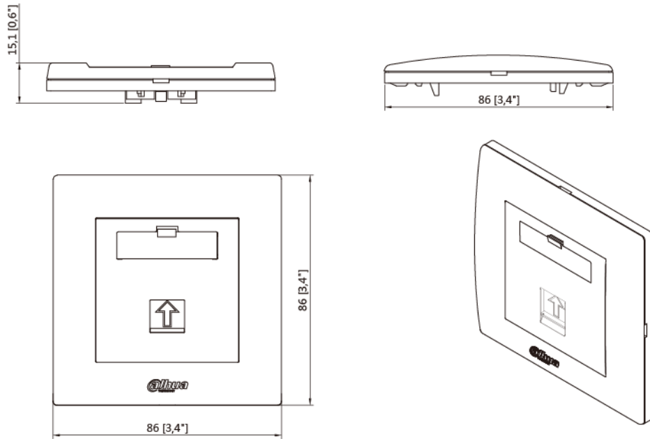
DH-PFM971-1_dimension
